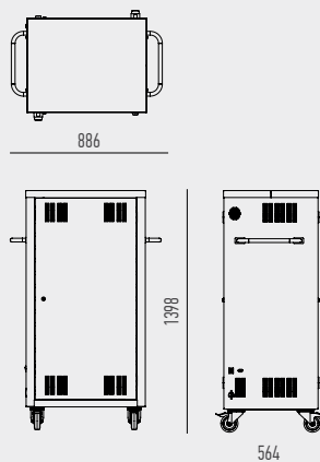
NBUS 16 / NBUS 32
