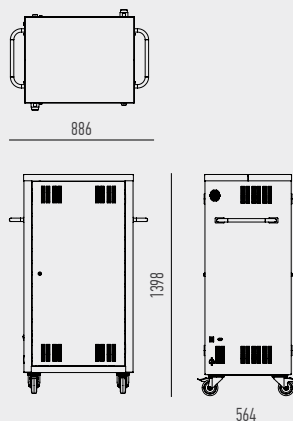
NBUS 16 / NBUS 32
