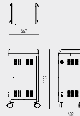
NBUS 30T
