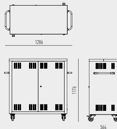
NBUS 30 / NBUS 40
